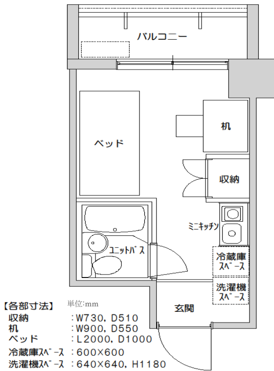
《A棟居室平面図》
